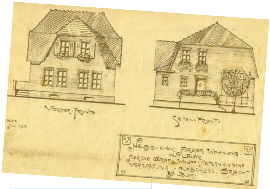
Liblar, Carl-Schurz-Str. 65, Entwurfszeichnung des Mauermeisters Gottfried Popp (Lechenich) für das neue Forsthaus, 1913 (StAEft, Best. D 03/1 – Erfurt 50, Bl. 26)
